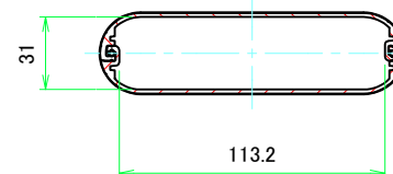
A-A (1:2.5)
